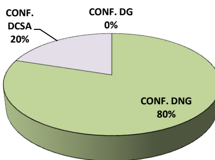
Dengue confirmado
