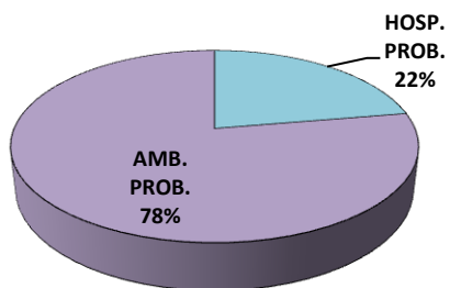
Hospitalizado/Ambulatorio probables
