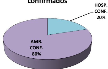
Hospitalizado/Ambulatorio confirmados
